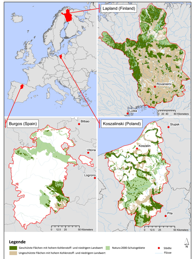
Abb. 2: Gebiete mit hohem Bodenkohlenstoffanteil und niedrigen Landpreisen innerhalb und außerhalb europäischer Natura 2000-Schutzgebiete
